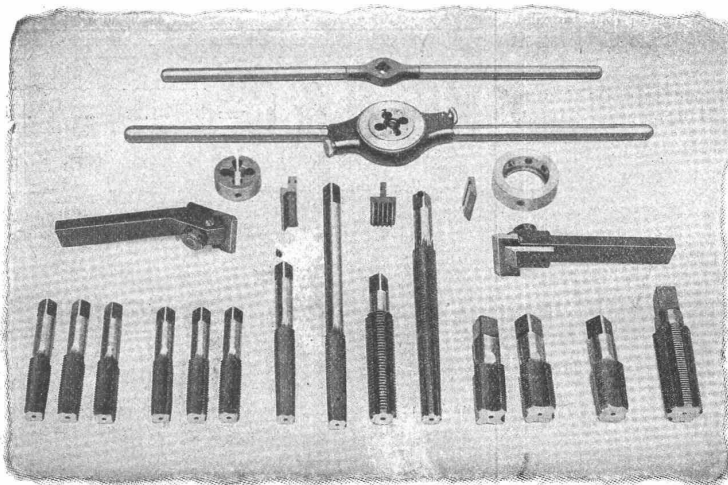
Gruppe von Gewindeschneidwerkzeugen.
