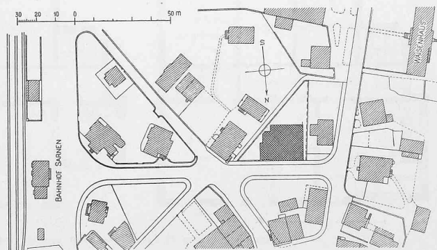
Lageplan. — Masstab 1:2500.
