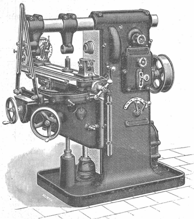
Wanderer-Rapid-Fräsmaschine Nr. 2 mit Einzelscheiben-Antrieb.
