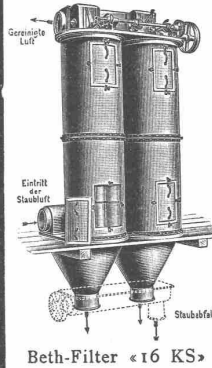
Beth-Filter «16 KS»
