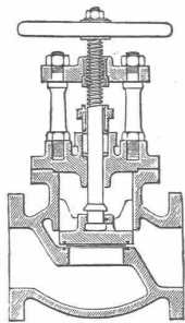
Stahlguss-Ventile mit Patendichtung.
