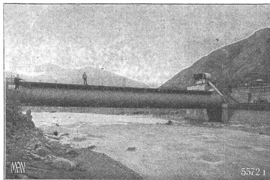
Walzenwehr.
