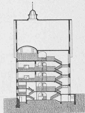
Schnitt. — Masstab 1:800.
