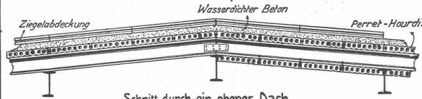
Schnitt durch ein ebenes Dach
