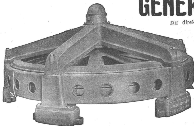
1/2 natürl. Grösse Drehstromgenerator 100 KVA, 7500 Volt, 50 Cycles, 40 Touren, für Bremen
