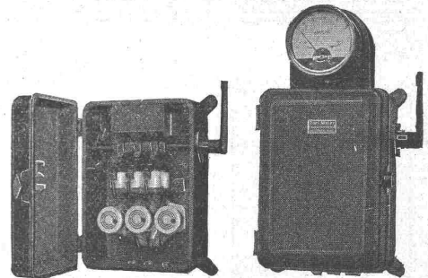
Motorschaltkasten Type KTM , 250 Volt, 40 Ampère, 500 Volt, 25 Ampère.
