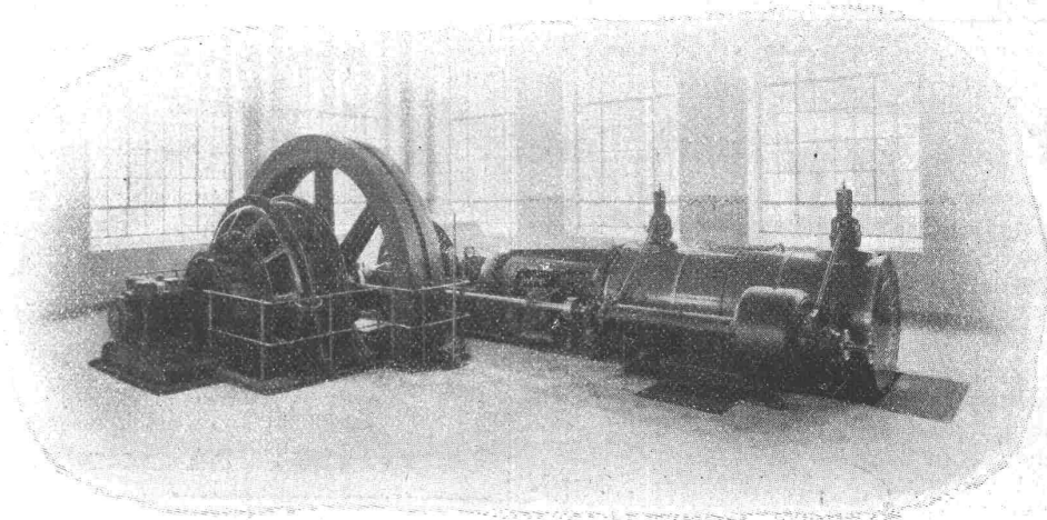
700 PS-Gleichstrom-Dampfmaschine im Guss- und Armaturwerk Kaiserslautern.
