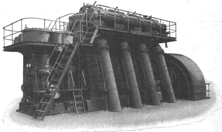
2400 PS-Sulzer-Diesel-Zweitaktmotor.
