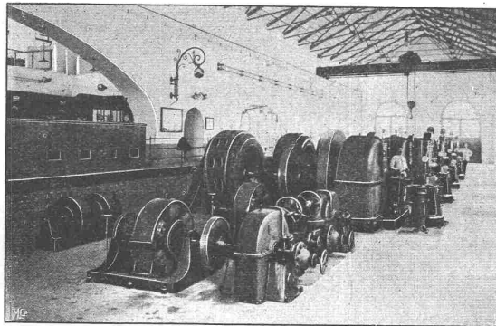
Usine des Farettes, près Aigle (Vaud).
