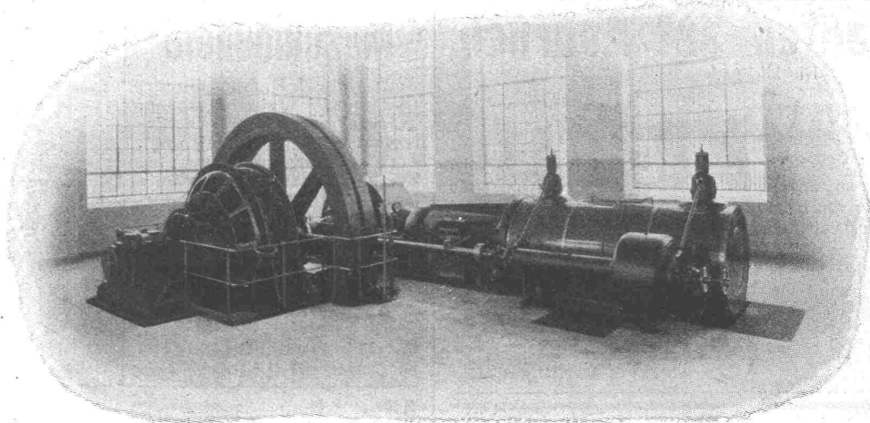
700 PS-Gleichstrom-Dampfmaschine im Guss- und Armaturwerk Kaiserslautern.
