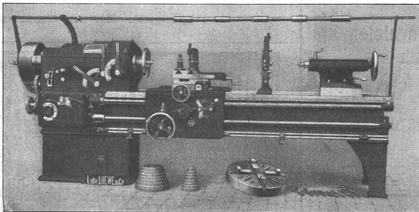
Leitspindel-Drehbank mit Einscheiben-Antrieb Nr. 3 Cc.
