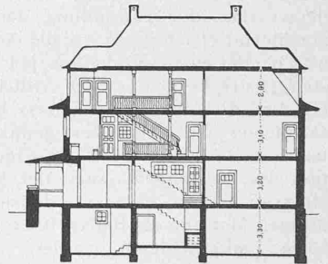
Abb. 5. Längsschnitt. — 1 : 400.
