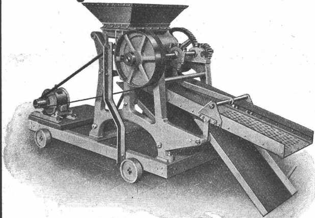
Fahrbarer Kohlenbrecher mit elektrischem Antrieb.
