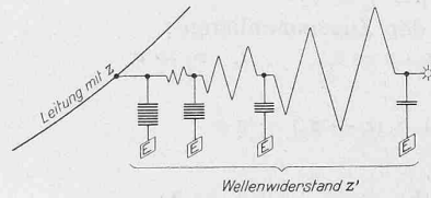
Abb. 3. Reflexionsfreie Brandung von Ueberspannungen.
