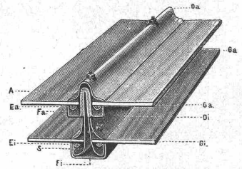
b) Duplexsprosse.
