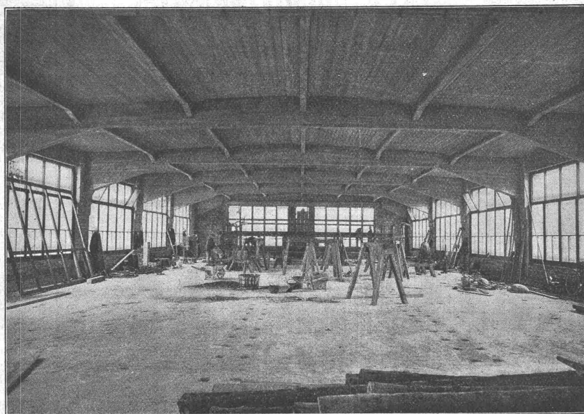
Stickerei-Neubau, Dachkonstruktion über dem Maschinenaal mit 18 m Spannweite.
