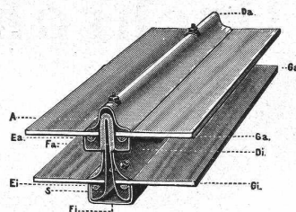
b) Duplexsprosse.
