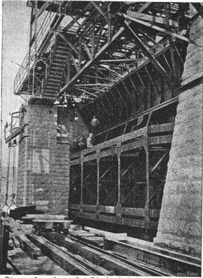
Stauwehranlage im Rhein bei Augst-Wyhlen. (Schützen 9 × 18.5 m Größe).
