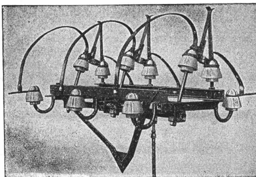
Freileitungsschalter
