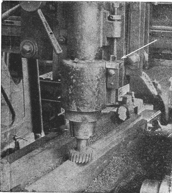
Obige Figur zeigt die Anwendung von Loewe'schen Parallelendmassen , um auf einer Fräsmaschine zwei Flächen in gegebenem genauen Vertikal-Abstand von einander zu bearbeiten. Der Pfeil zeigt die Lage des Endmasses.
