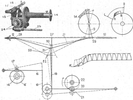
Spinnregler und schematische Darstellung des Reguliervorganges.
