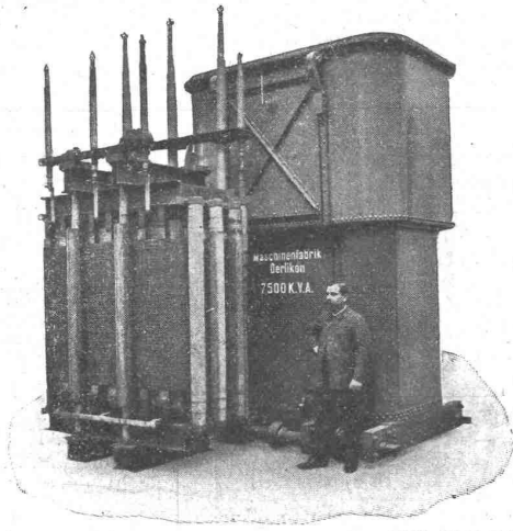
7500 kVA-Drehstrom-Öltransformator für 8650/60.000 Volt.
