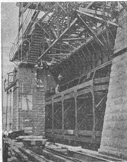
Stauwehranlage im Rhein bei Augst-Wyhlen (Schützen 9 x 18,5 m Grösse).
