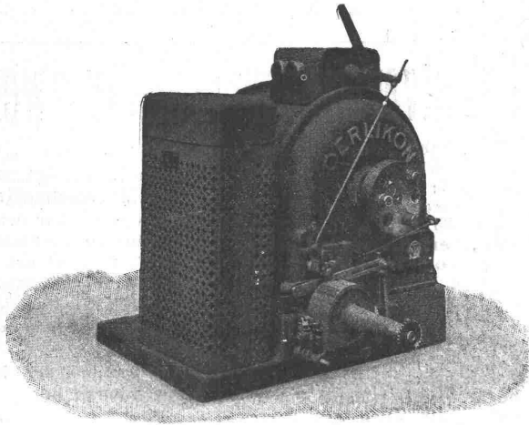
Drehstrom-Kollektormotor für Ringspinnmaschinen-Antrieb.
