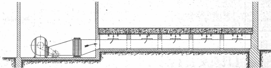
Trockenanlage mit Sendric-Apparat und Sulzer-Zentrifugal-Ventilator. Leistung: Erwärmen von 20000 m 3 Luft pro Stunde von 0 auf 90° C.
