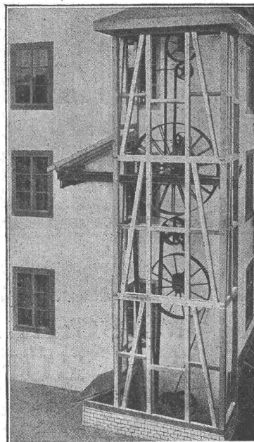
Umänderung einer stehenden Welle mit konischen Rädern in vertikale Lenix- Rientriebe in einer Baumwollweberei
