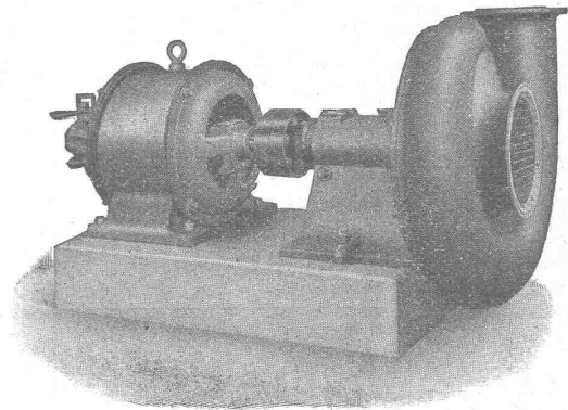
Einstufiger Hochdruck-Zentrifugalventilator
