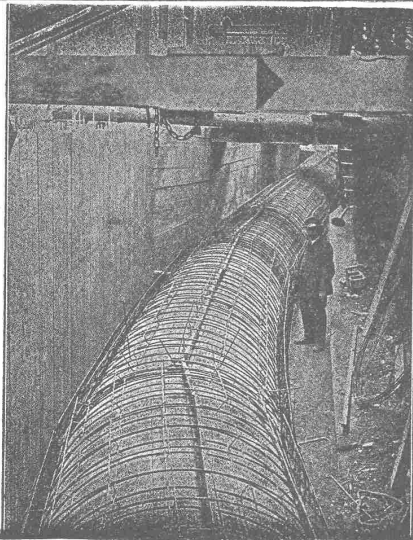
Druckrohr in Eisenbeton von 2 m Durchmesser der Wasserkraftanlage Stöckli & Cie., Basel, 1916/17.
