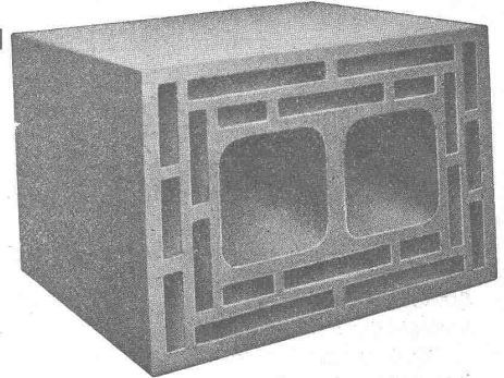
Das beste, billigste Rauchkamin.
