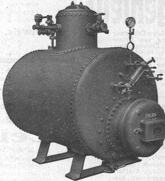
Elektrischer Dampfkessel für 120 kW Aufnahme
