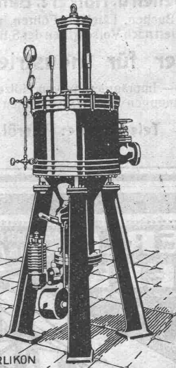
Elektroden-Dampfzerzeuger, Syst. Revel, 500 kW
