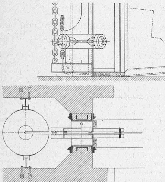
Abb. 19. Rahmenfuss zum Abschluss-Vorhang, darunter: Horizontalschnitt. — Masstab 1:30.
