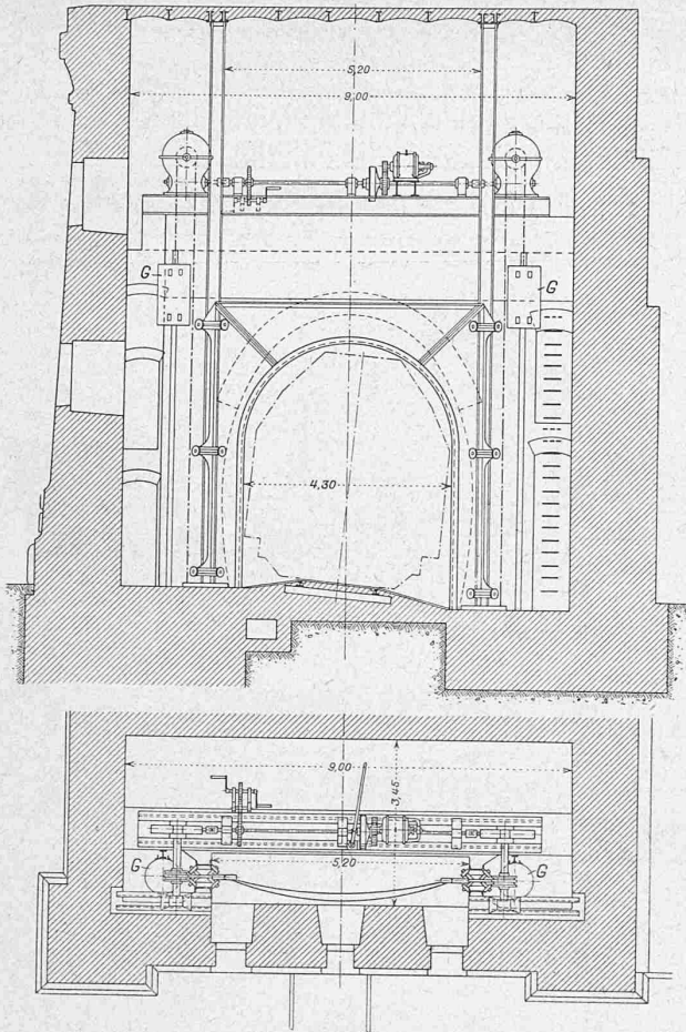
Abb. 18. Abschluss-Vorhang am Tunnelportal. — 1:150.
