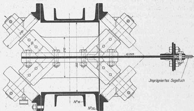
Abb. 20. Führungsrollen des Vorhang-Rahmens. — 1:10.
