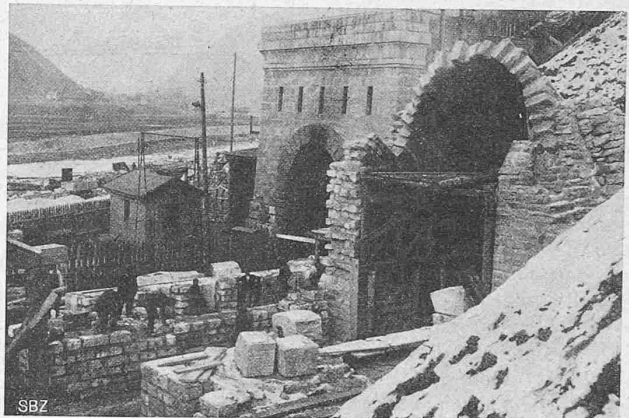
Abb. 16. Portal II im Bau, rechts „Pfeife“ zu Tunnel II.
