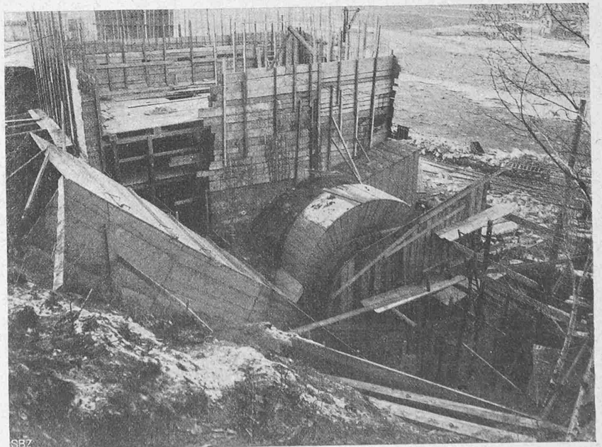
Abb. 13. Verschaltung des Ventilatorenhauses (vergl. auch Abb. 14).
