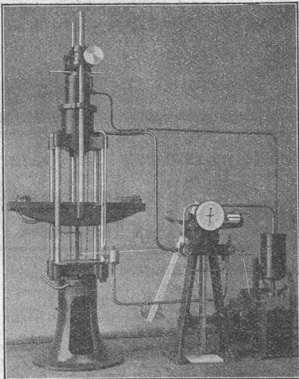
30 tons Zerreismaschine
