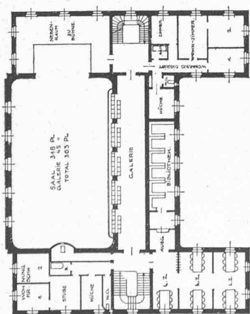
Grundrisse. — Masstab 1 : 600.
