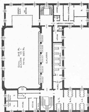
Grundrisse. — Masstab 1 : 600.
