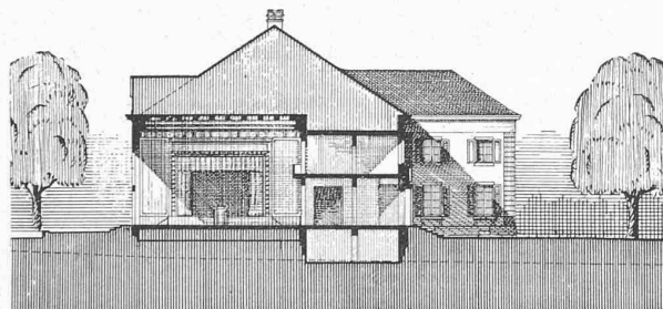
Querschnitt 1 : 600.
