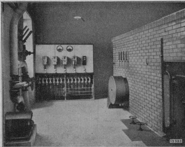
Elektrische Heizanlage in der Broncewarenfabrik A. G., Turgl. Anschlusswert 135 kW, Gesamt-Speichervolumen 15 m 3 , einschl. Inhalt des alten Heizkessels. Feinregulierung.
