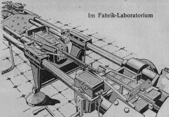
Drahtseil-Zerreiss-Versuch
