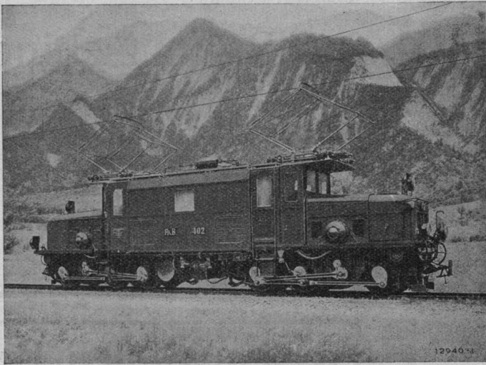
Einphasen-Schnellzugslokomotive mit Einzel-Achsantrieb Type 2-C-1 für die Schweizerischen Bundesbahnen, 3 \times 700 PS, 15000 Volt Fahrdrachtspannung, 16\frac{1}{3} Perisee, max Geschwindigkeit 60 bis 90 km/h.
