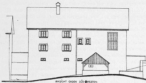
ANSICHT GEGEN SÜDWESTEN.
