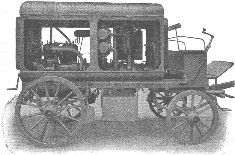
Fahrbare Kompressor-Anlage
