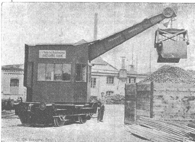
Lokomotivdrehkran mit Akkumulatorenbetrieb, 5 Tonnen Tragkraft, im Rheinhafen Basel.
