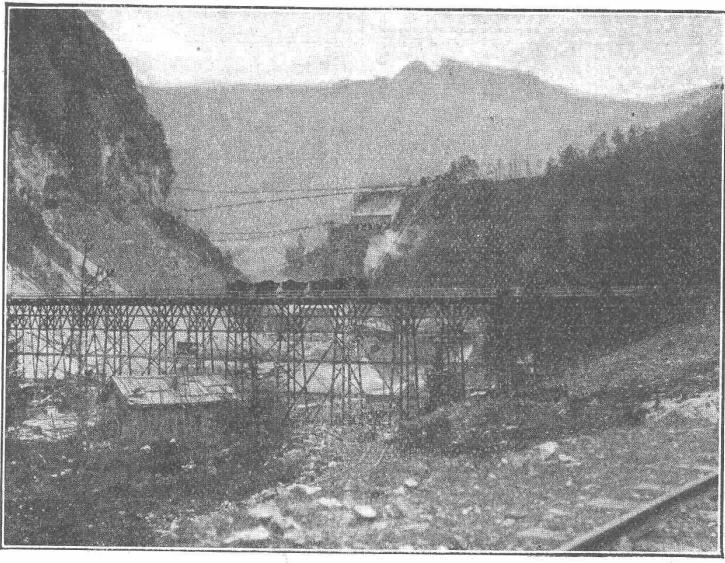
Staumauer Schräb :: Dienstbrücke zwischen Kilchblatt und Aufbereitung. Bauausführung gemeinsam mit Ed. Züblin & Cie. A.-G.
