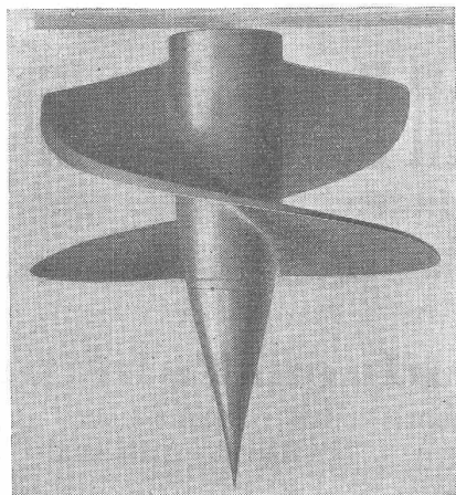
Lauf- rad einer Bell-Schnellläuferturbine für spezifische Drehzahlen von 700-1100 per Minute.
