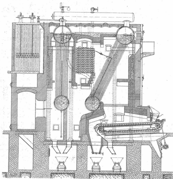
Sulzer-Steilrohrkessel (Patentiert)
