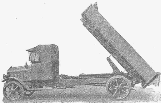
Dreiseiten-Motorkipper
