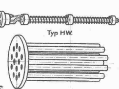
Einzelne elektrische Heizsätze zum Einbauen.
