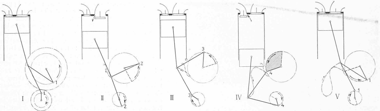
Viertaktmotor von Andraeu mit ungleichen Hüben. — Schematische Darstellung der einzelnen Kolben-Endstellungen.
