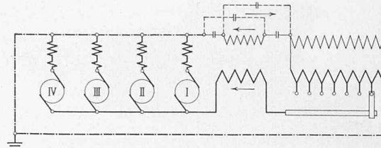
Abb. 4. Schaltung des Transformators bei der A^{e\frac{4}{6}1} -Lokomotive.
