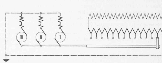
Abb. 3. Schaltung des Stufentransformators der A^{e\frac{3}{6}1} -Lokomotive.
